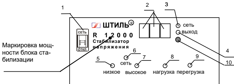
Рисунок 4.1 Передняя панель блока стабилизации
